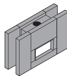
Cheminée à poser DF7
